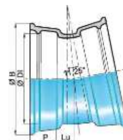
DN 350-600
