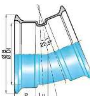
DN 250-300
