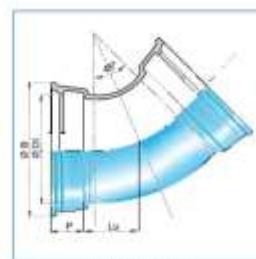
DN 350-600
