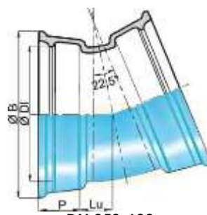
DN 350-600
